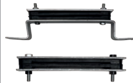
Kasnak Muhafazası AZZ - YP43 Pulley Cover AZZ - YP43
